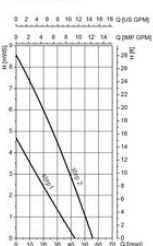
FP 314 PP-32/25 FP 314 S-28/25
