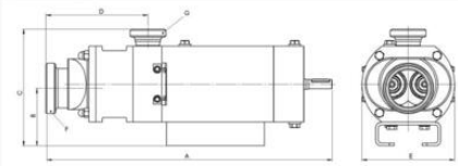
Måle HTGASPN H1 axel (mm)
