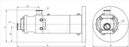
Måle HTGASPN komplettmotor (mm)
